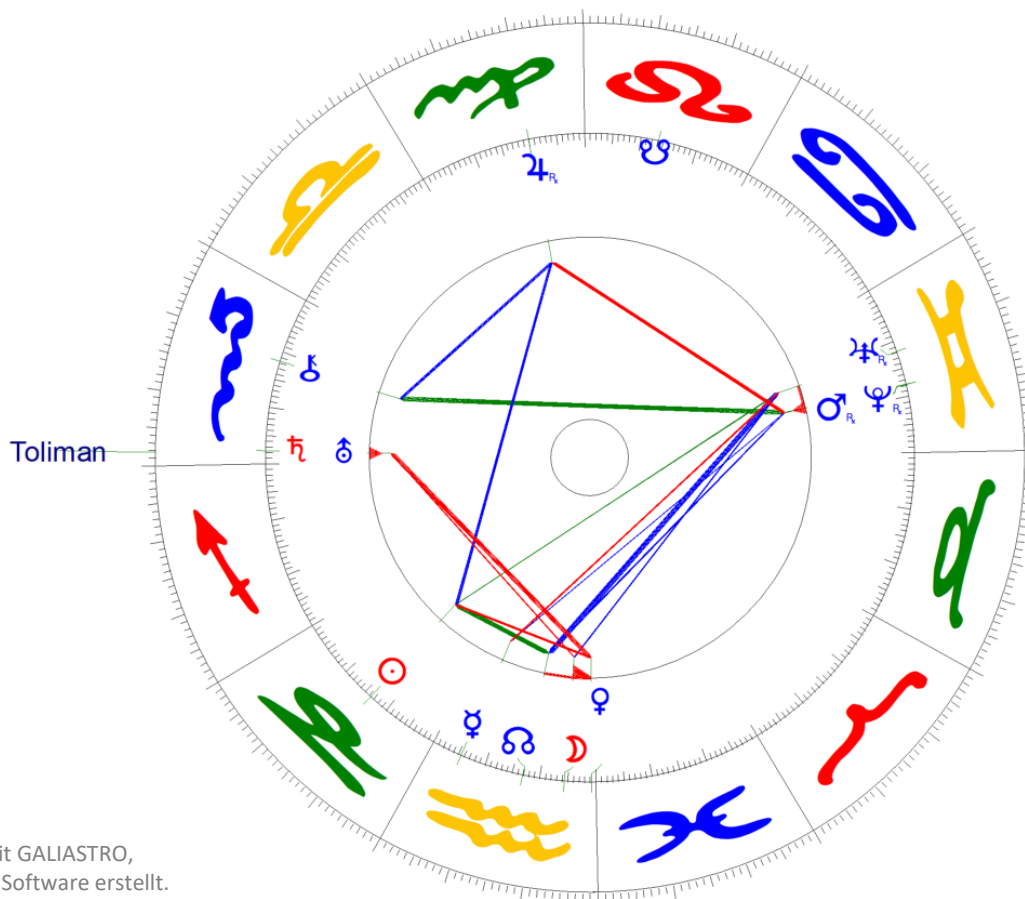
Saturn/Uranus-Konjunktion am 06.01.1897 in der Nähe des Fixsterns Toliman
